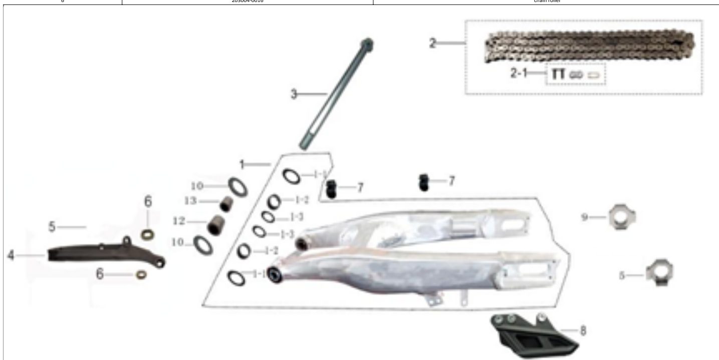
平叉组件
