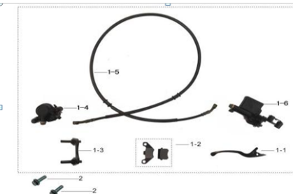
后制动总成
