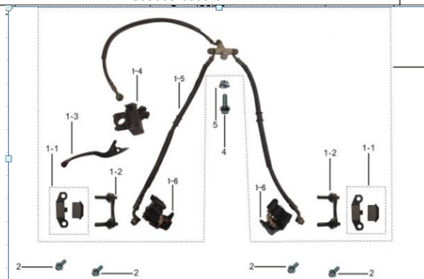
前制动总成
